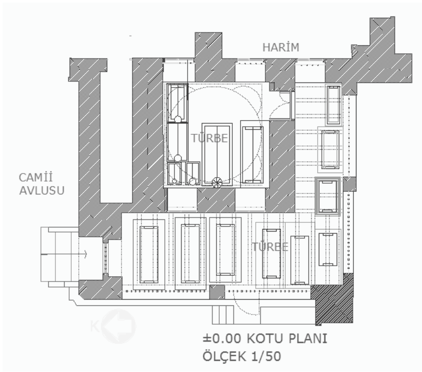
Çizim 5: Sahabeler Türbesi'nin Planı (VBM'den İşlenerek)
